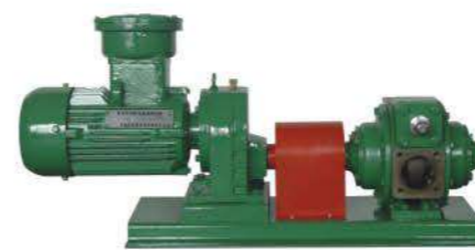
联轴器传动 Coupling Drive
